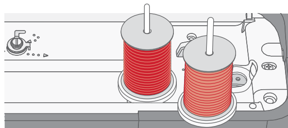
Broche porte-bobine repliable et broche porte-bobine principale en position verticale.
